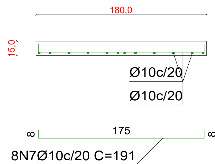
Seção B-B
