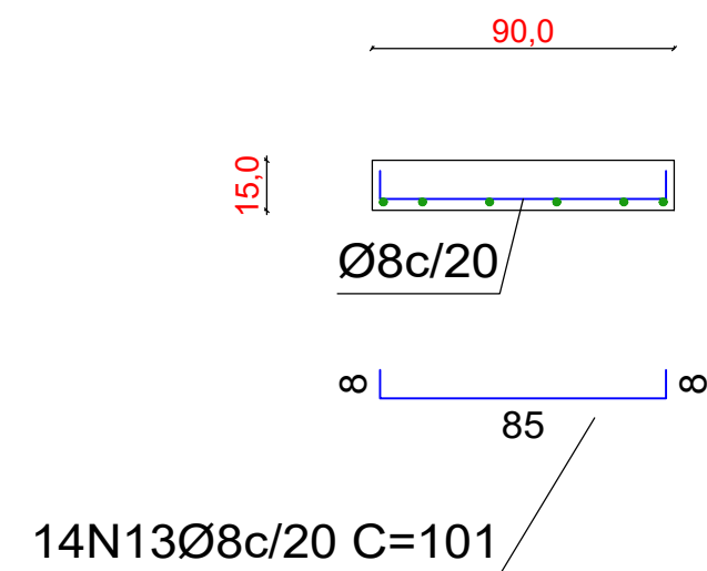
Seção E-E
